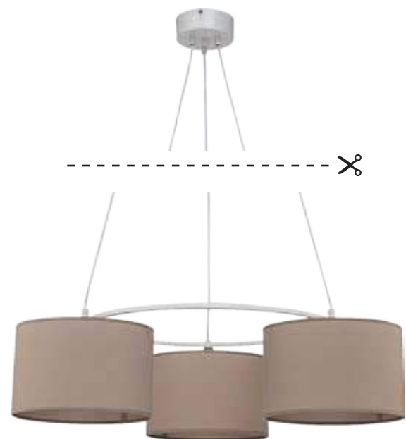
8261 TEQUILA ↑ max 120 cm ↔ 70 cm ⚡ 3 x E27 max 40W
