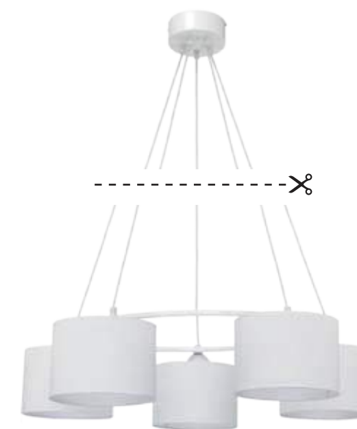
8263 MARGHERITA ↑ max 120 cm ↔ 65 cm ⚡ 5 x E27 max 40W
