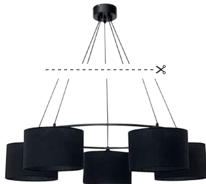
8244 TEQUILA ↑ max 120 cm ↔ 100 cm ⚡ 5 x E27 max 40W
