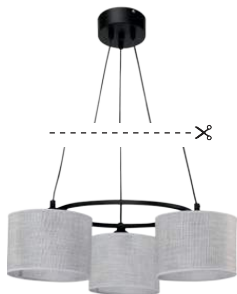
8270 MARGHERITA ↑ max 120 cm ↔ 45 cm ⚡ 3 x E27 max 40W
