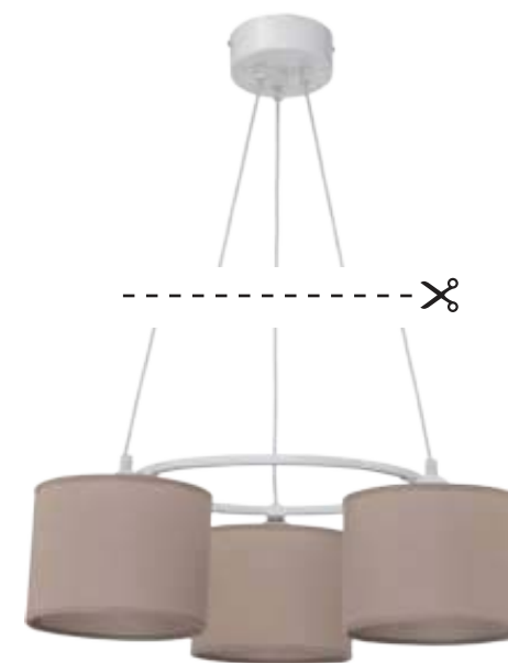
8266 MARGHERITA ↑ max 120 cm ↔ 45 cm ⚡ 3 x E27 max 40W
